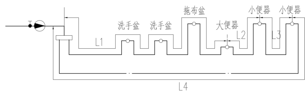
图 1 男卫生间配水管环状连接示意图
