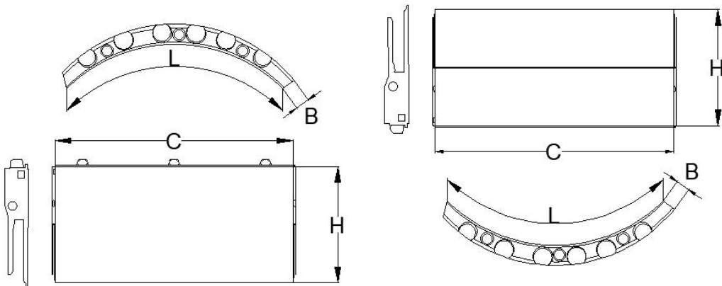
图 A.0.1 圆形管道标准段管片构造示意图
