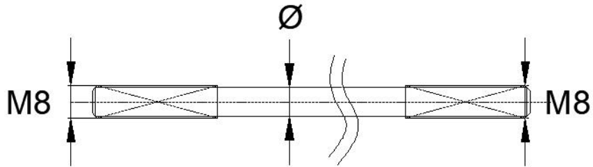
图 B.0.1 长螺栓尺寸
