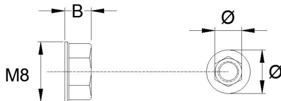
图 B.0.4 M8 螺帽
