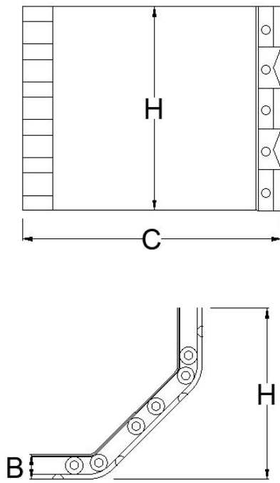
图 A.0.4 非圆形（矩形）管道角隅部件
