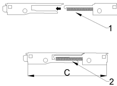
(c) 有抗震要求的调整用部件剖面示意图
