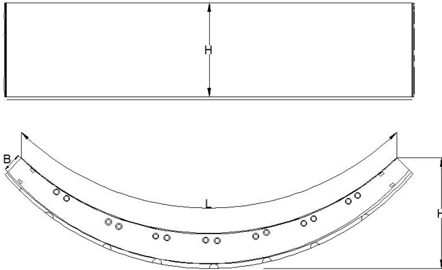
图 A.0.1 圆形管道标准段管片构造示意图
