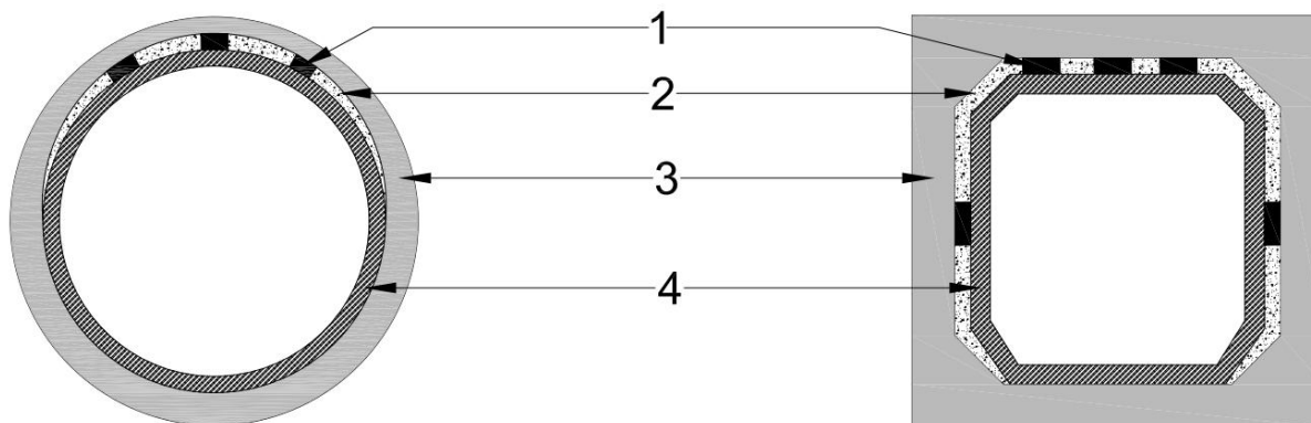
图 4.1.3 管片内衬法结构
