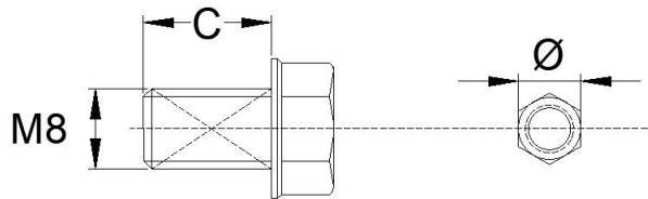
图 B.0.3 M8 短螺栓
