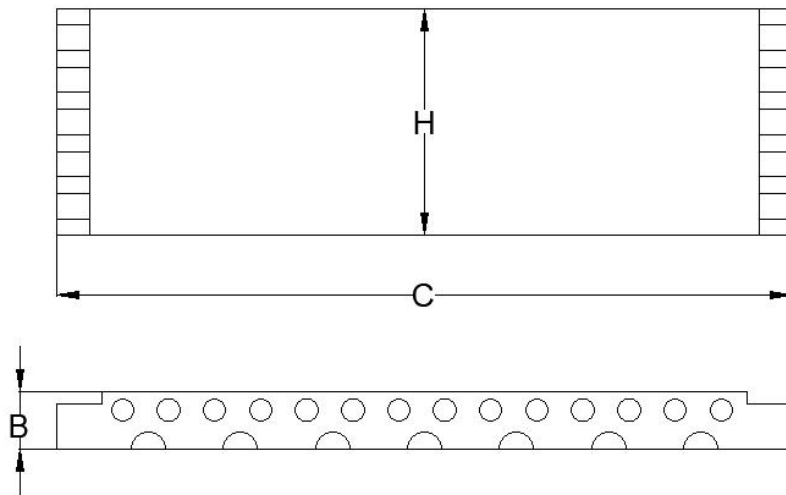
图 A.0.3 非圆形（矩形）管道直线部件
