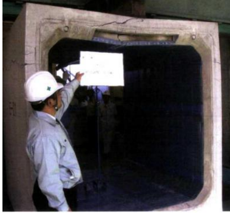
图3 矩形管外压试验状况
