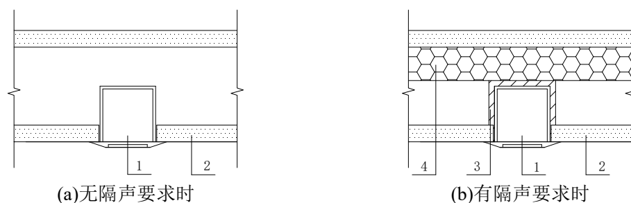
图 4.5.3-1 电源插座盒安装示意
