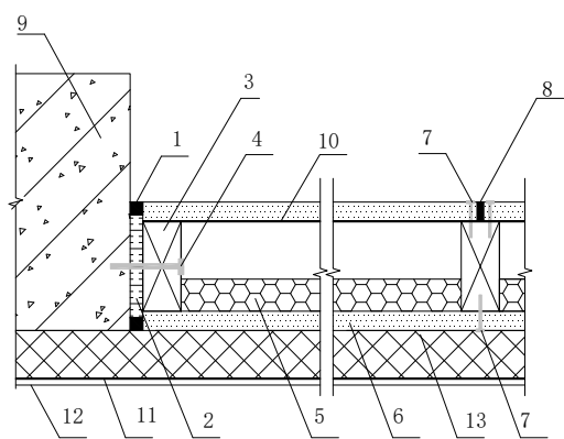
(b) 外墙（平齐式—有外保温层）
