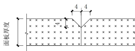
图 3 墙面板的倒角
