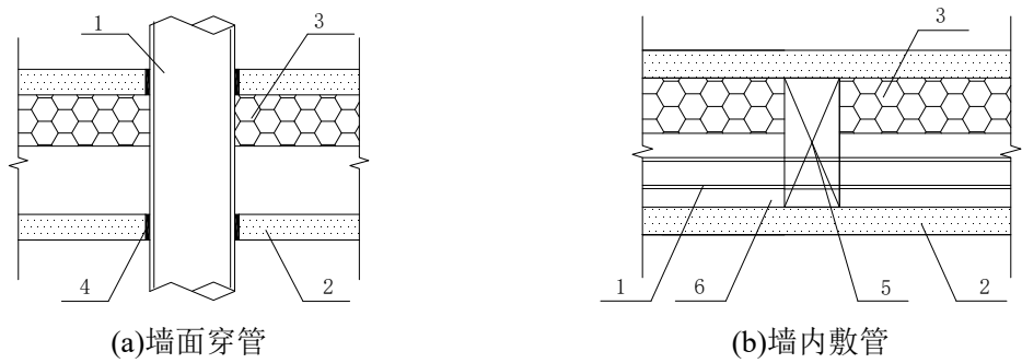
图 4.5.3-2 墙面穿管及墙内敷管安装示意
