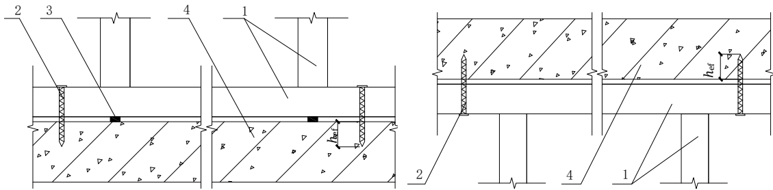
图 5.3.8 墙体与主体结构连接示意
