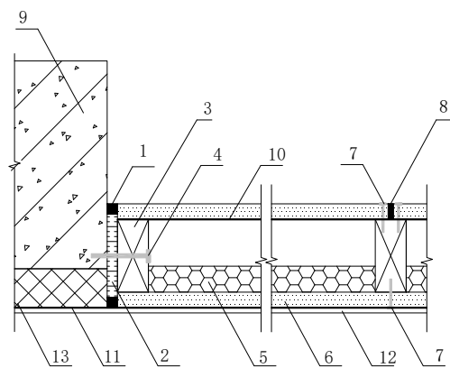
(b) 外墙（平齐式—有外保温层）
