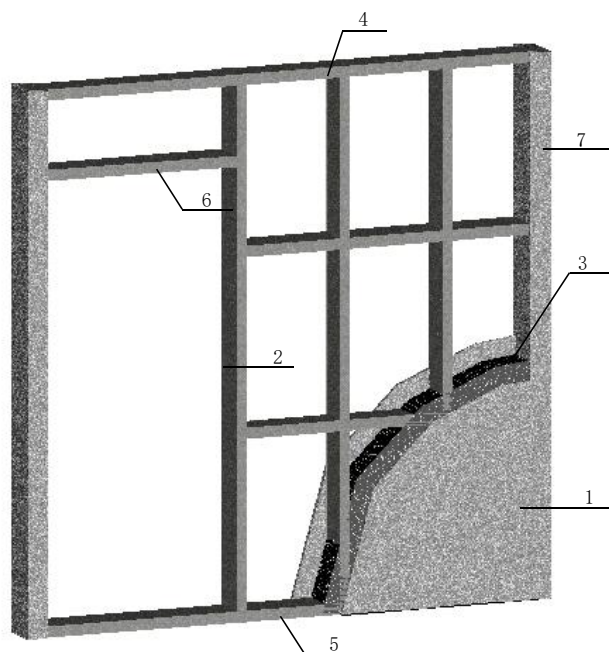
图1 竹基水泥板组合墙体构造示意图
