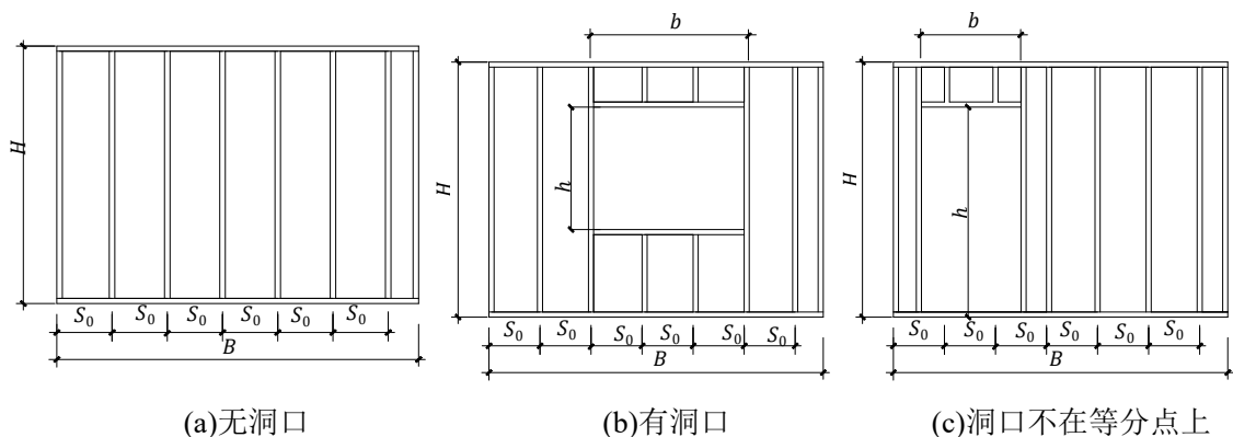
图 5.3.1 墙骨架布置示意
